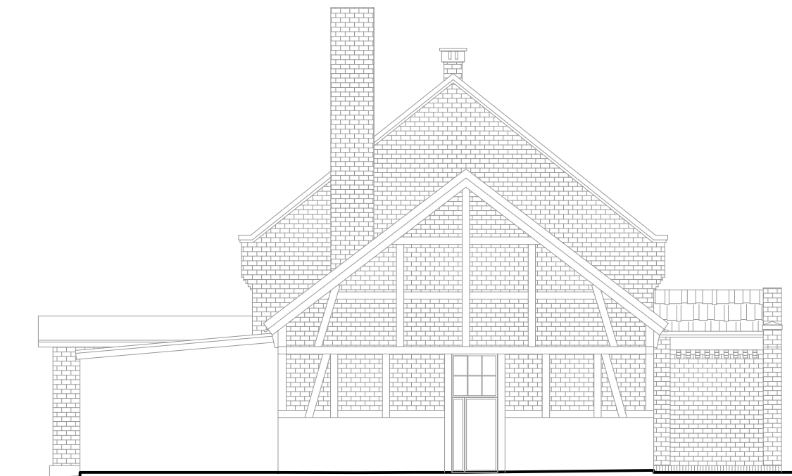
ELEWACJA FRONTOWA
