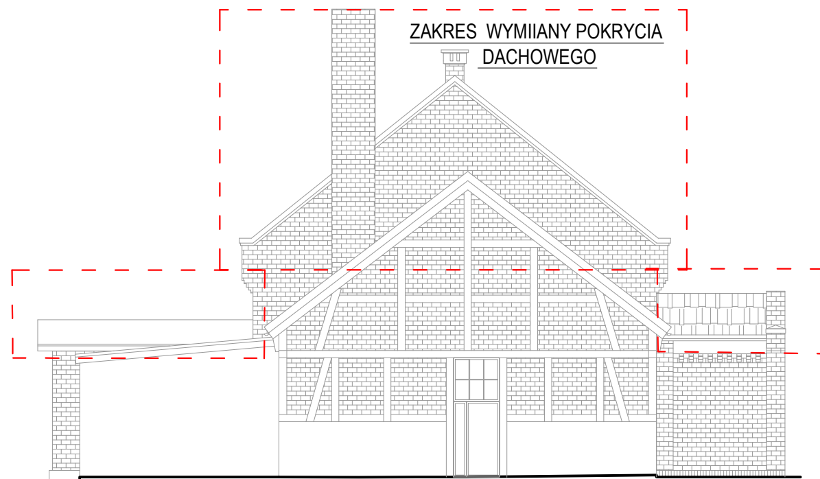
ELEWACJA FRONTOWA
